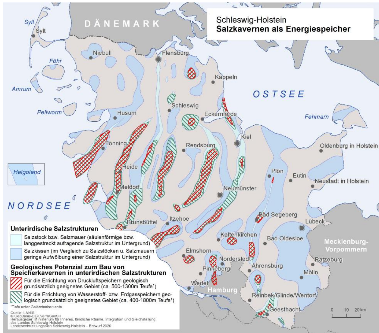
Themenkarte 13: Salzkavernen als Energiespeicher
