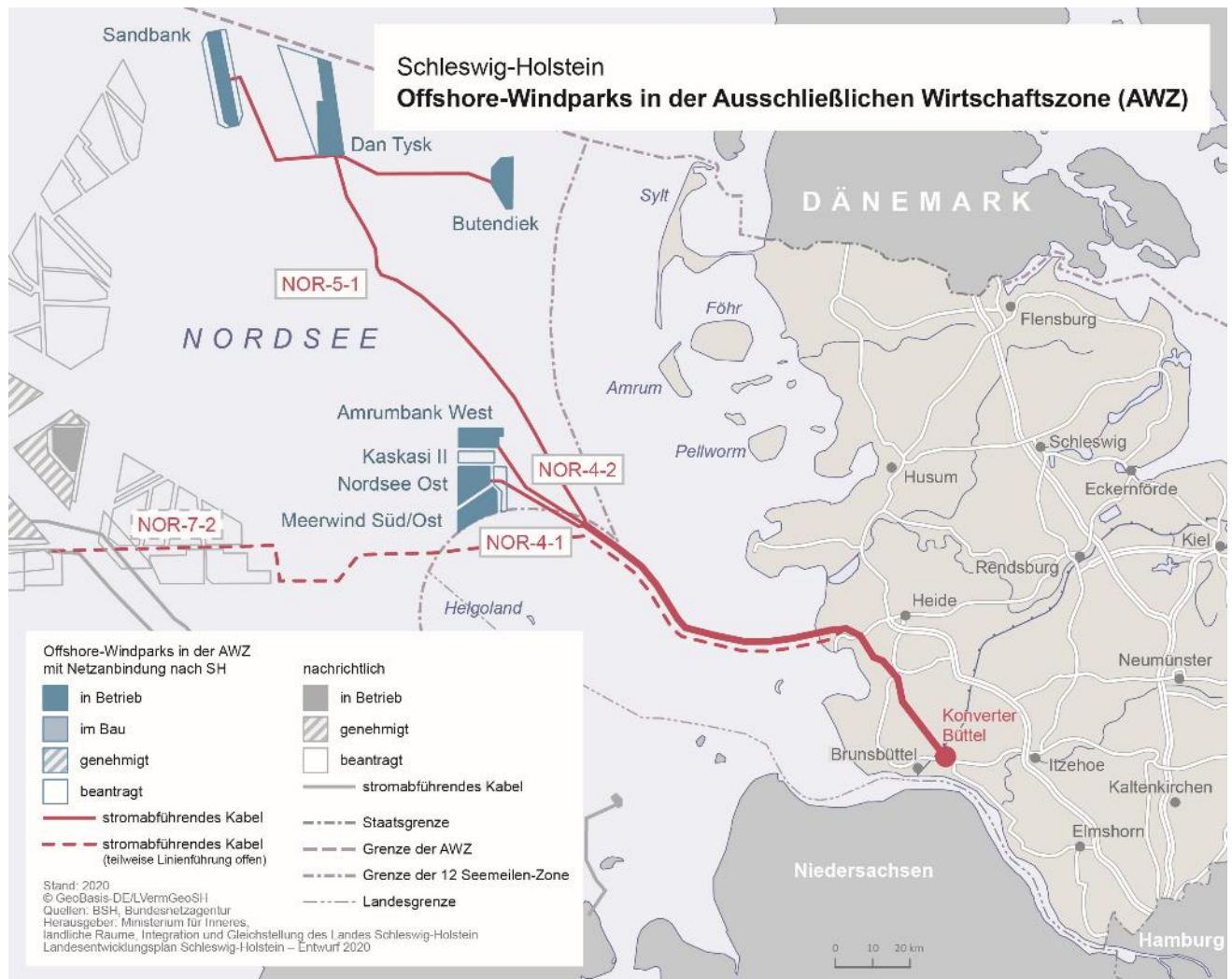
Themenkarte 15: Offshore-Windparks in der AWZ
